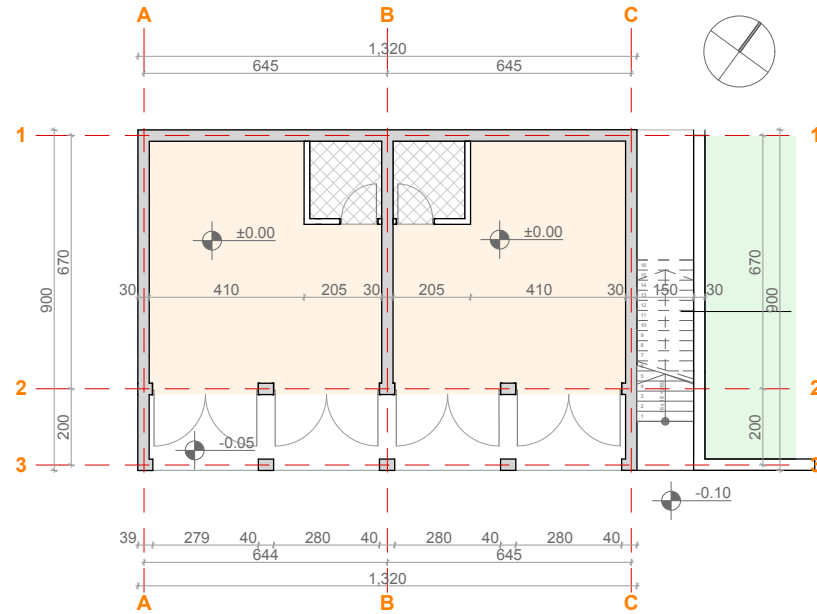
OSNOVA PRIZEMLJA
