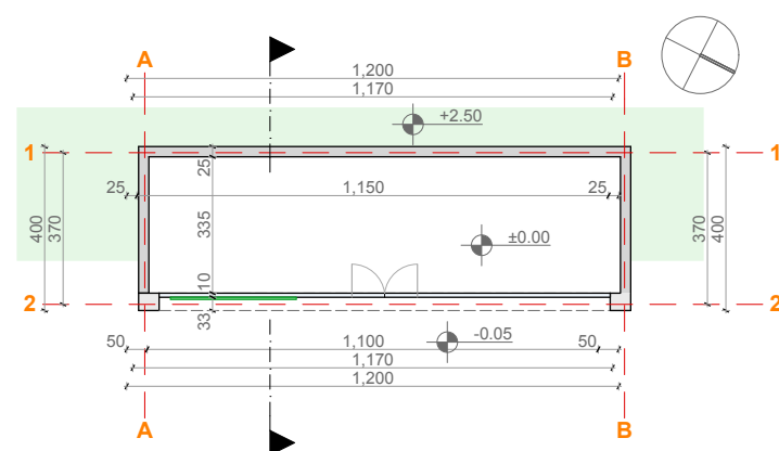
OSNOVA PRIZEMLJA
