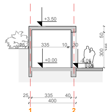
PRESJEK R
