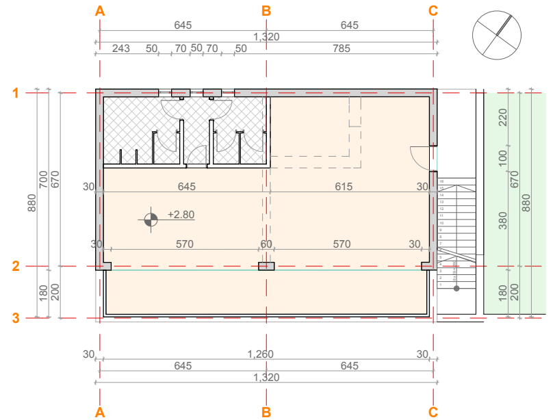
OSNOVA SPRATA
