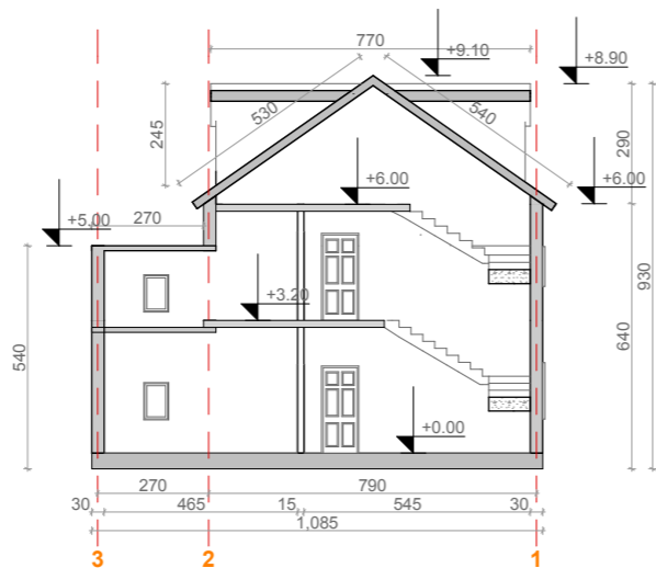
PRESJEK R
