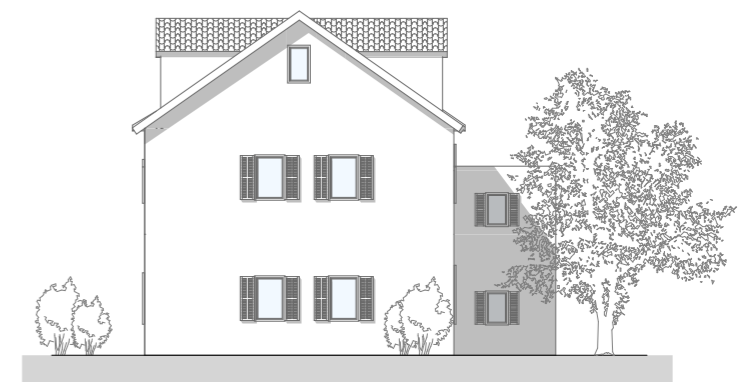
FASADA ZAPAD
