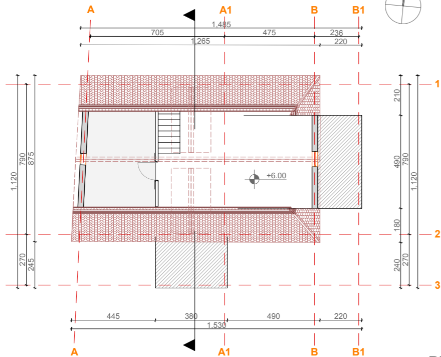
OSNOVA POTKROVLJA
