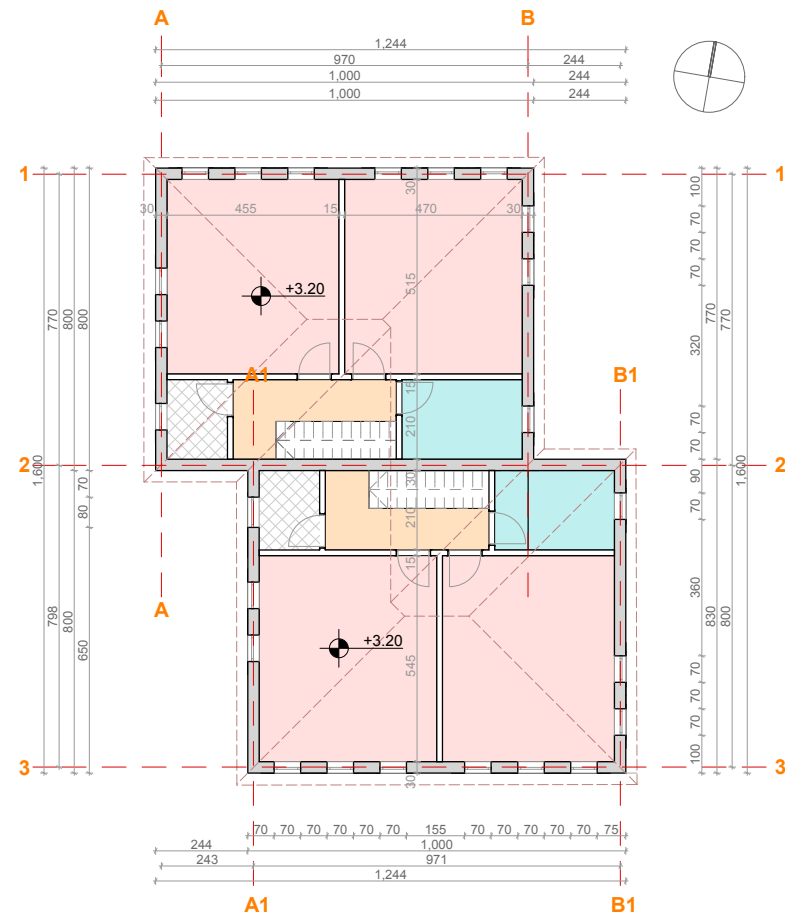
OSNOVA POTKROVLJA
