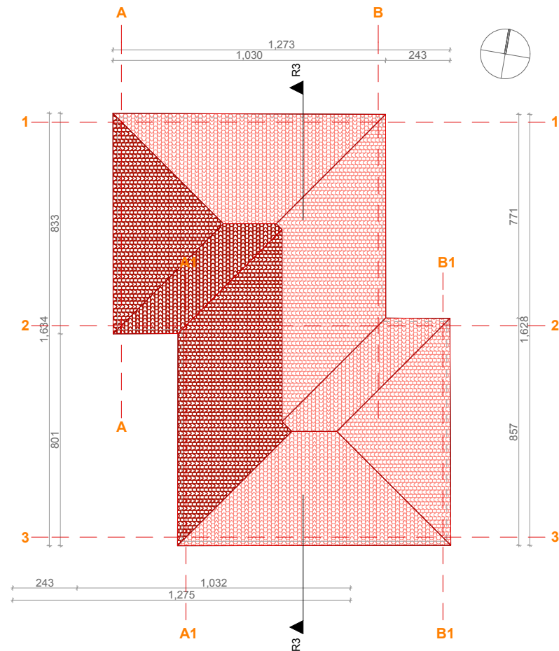
KROVNA RAVAN
