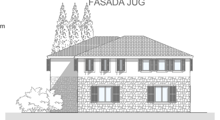
FASADA JUG
