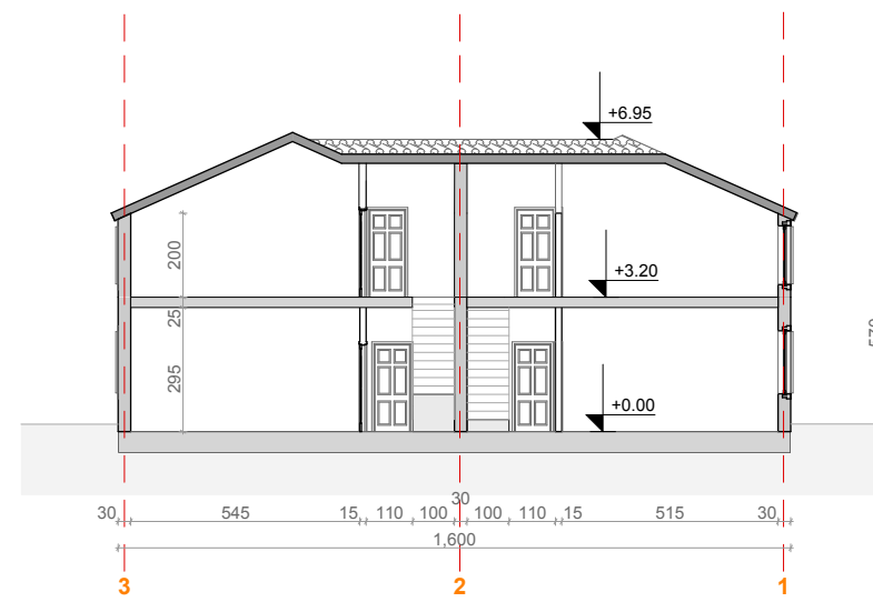
PRESJEK R
