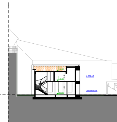
POPRECNI PRESJEK
