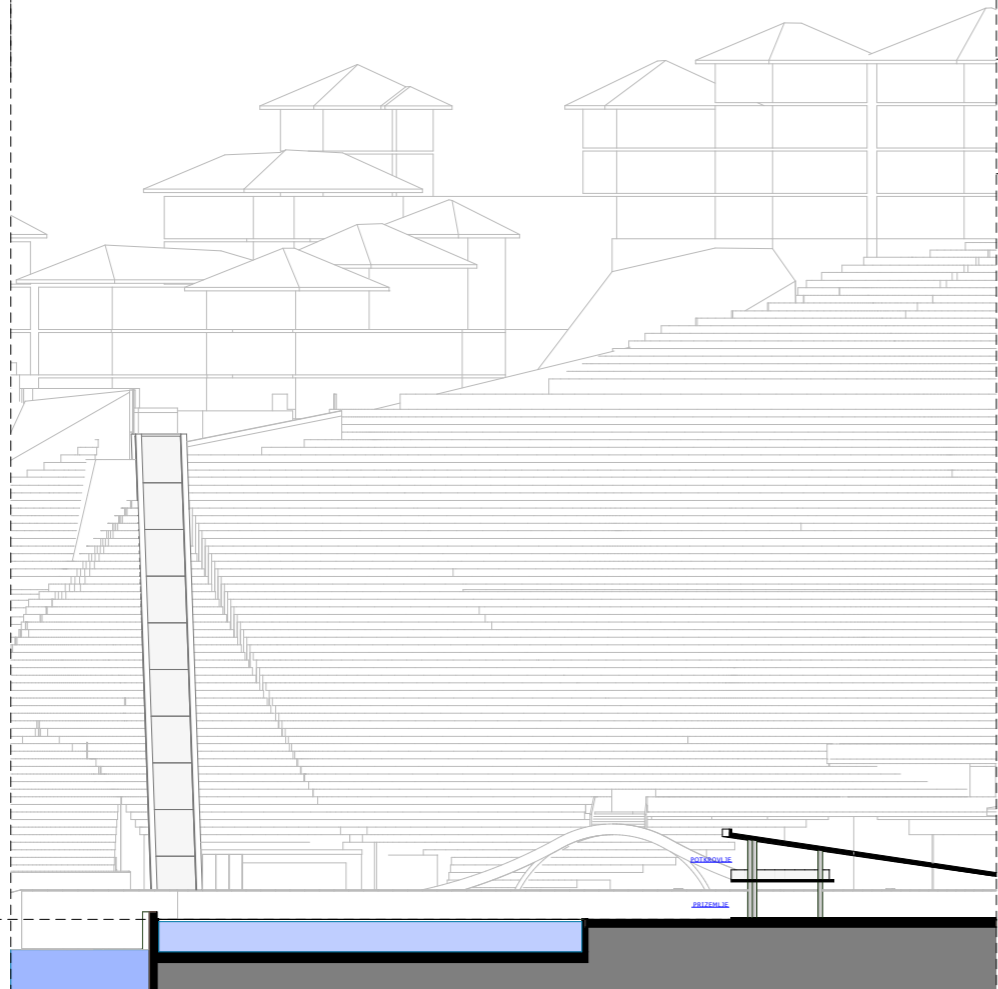
PODUZNI PRESJEK PLAZNOGA BARA I OTVORENOG BAZENA
