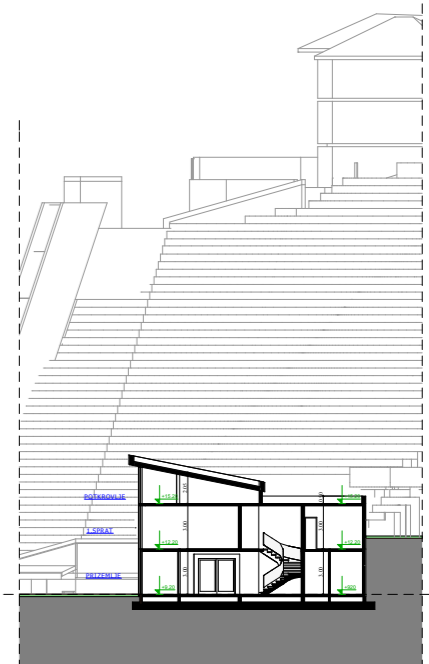
ZONA III PRESJECI 1:500
