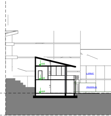
POPRECNI PRESJEK
