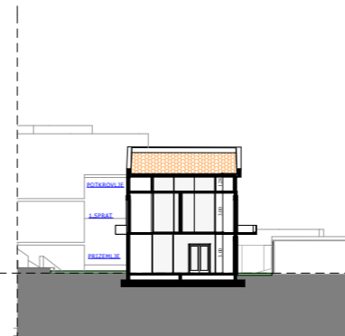
POPRECNI PRESJEK
