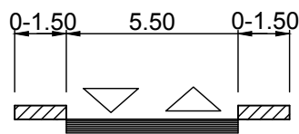
presjek 5 - 5
