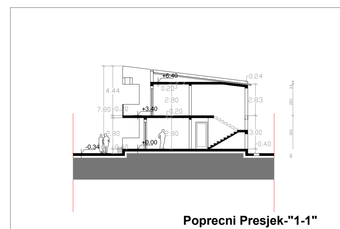
Poprecni Presjek-'1-1''
