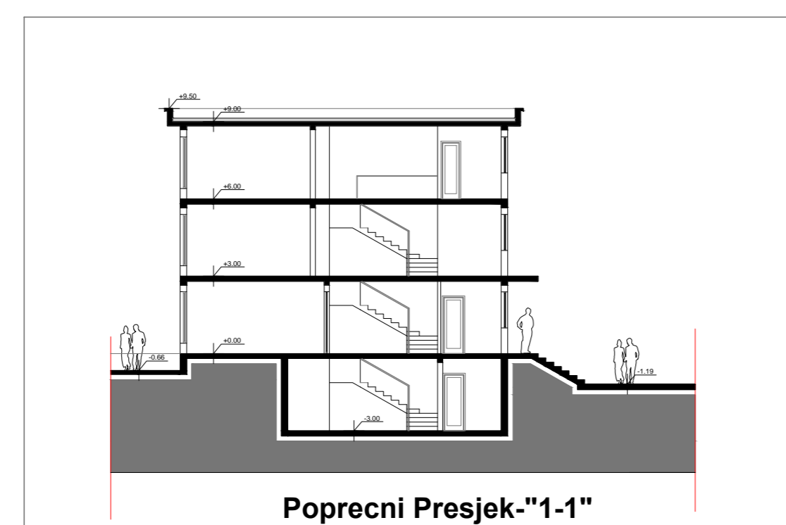
Poprecni Presjek-'1-1''
