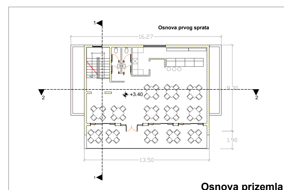
Osnova prizemlja
