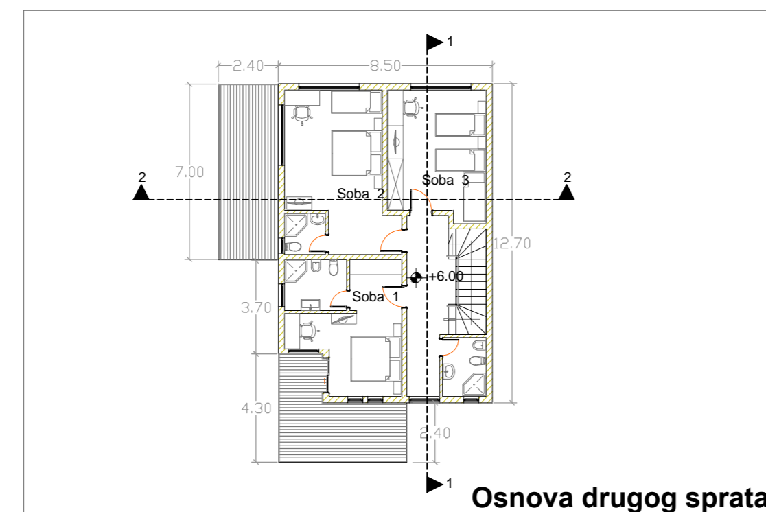
Osnova drugog sprata
