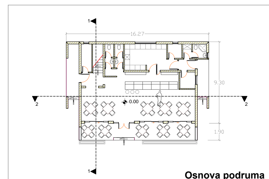
Osnova podruma
