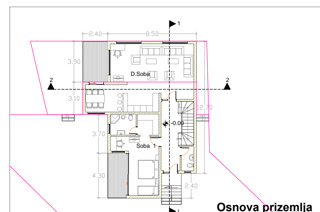
Osnova prizemlja
