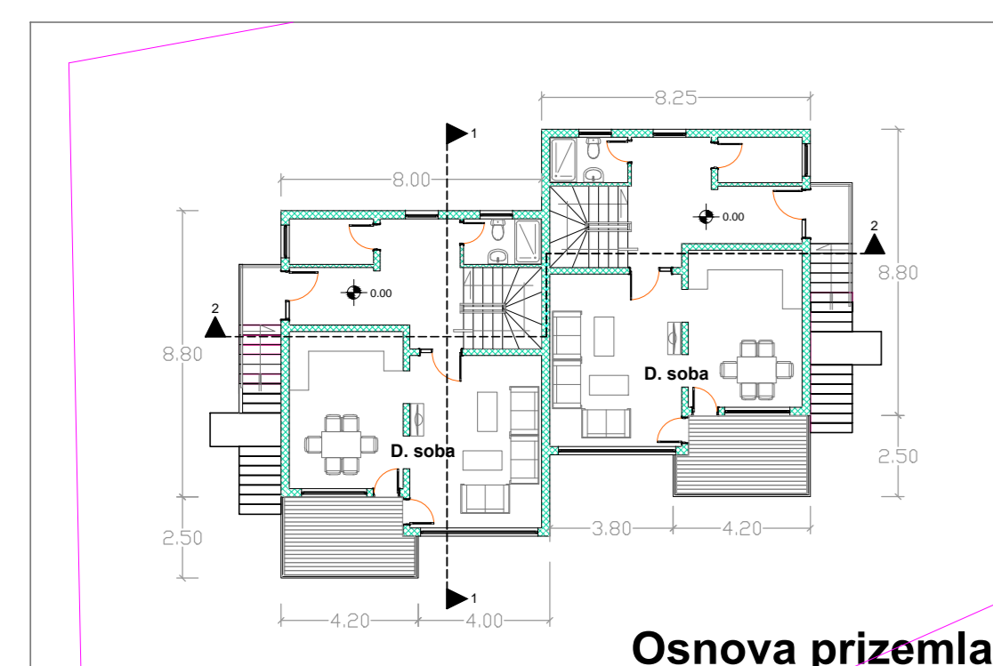
Osnova prizemla
