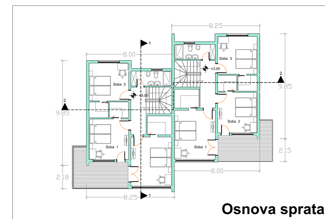
Osnova sprata
