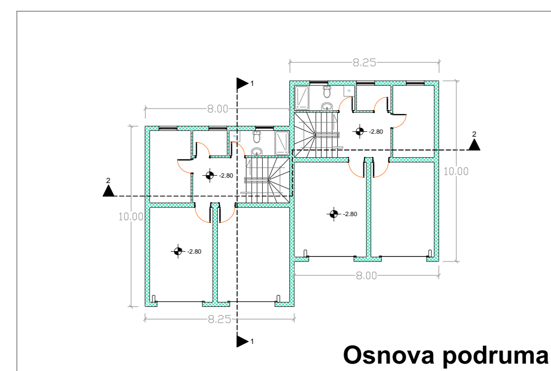
Osnova podruma
