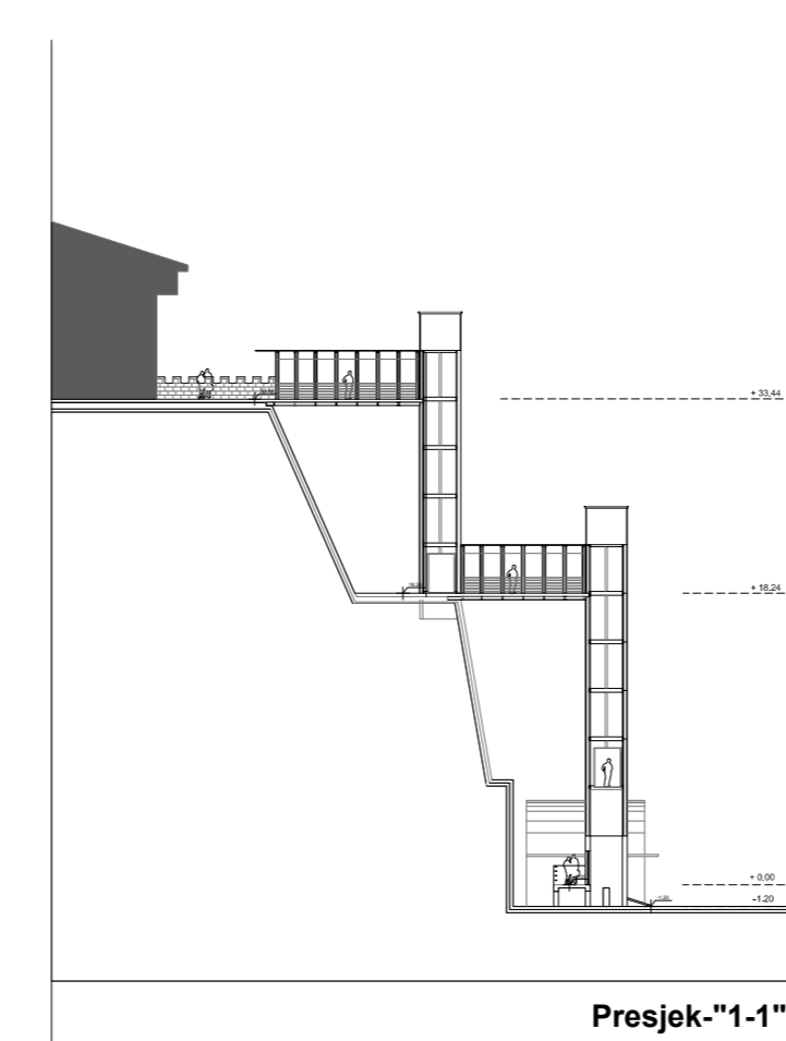
KARAKTERISTICNI PRESJECI KROZ OBJEKTE R 1 : 500
