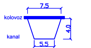
regulacija potoka Bratica
